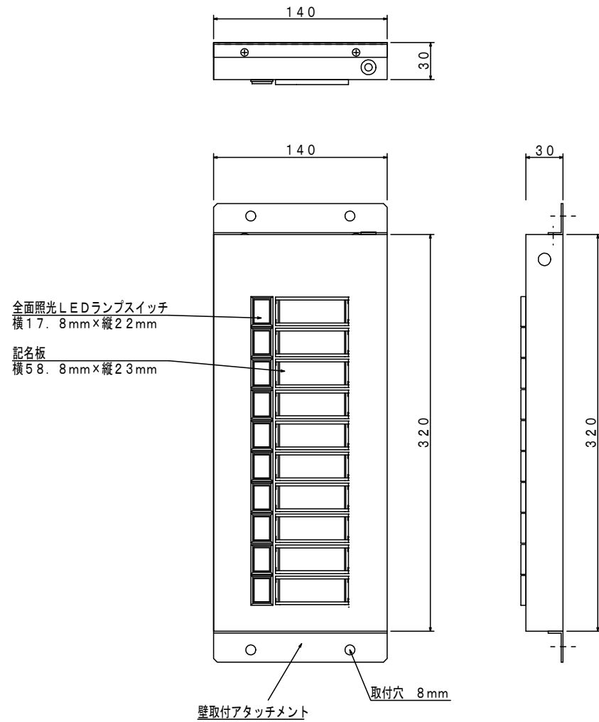
出退表示盤 C1A-10CH
