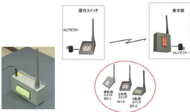
無線による表示システム (1)
